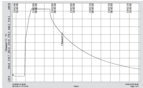
Rzeczywisty wykres z pieca procesu odprężania płyt Original stress relieving process example
